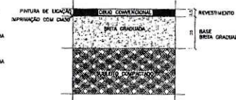
Perfil Estrutural Genérico do Pavimento Demais trechos de ruas
