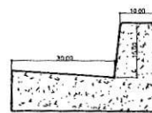
Detalhe Meio Fio e Sarjeta Moldado in loco Largura da Sarjeta= 0,30m
